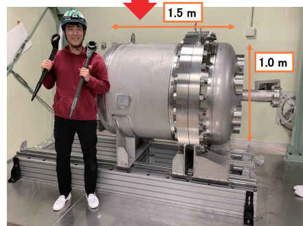
1000L検出器の圧力容器 @神岡鉱山地下
