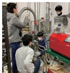
^3\text{He} , ^4\text{He} を用いた希釈冷凍機を用いた測定の準備
