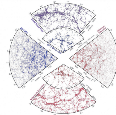
観測された銀河の分布(青)と 数値シミュレーション(赤)の比較
