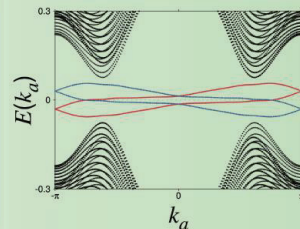
メビウス型トポロジカル超伝導の 表面状態
