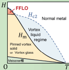
平行磁場下のFeSeの 磁場-温度相図 - Pauli常磁性が強い系の例 -
