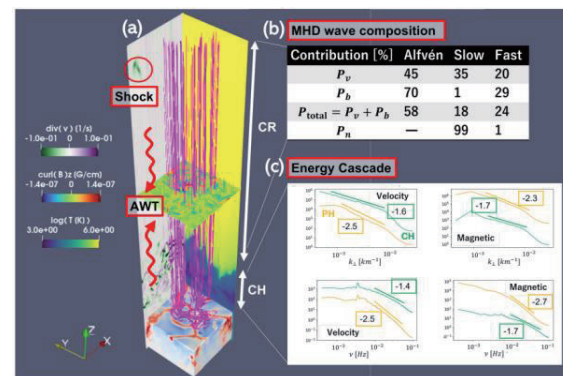
図4 太陽大気中での波動のカスケードとコロナ加熱(国吉2022、修士論文)
