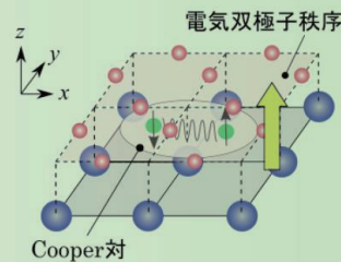
電気双極子秩序と超伝導の共存
