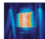
立方空間の中では超流動 ^3\text{He} はどうなるのか??
