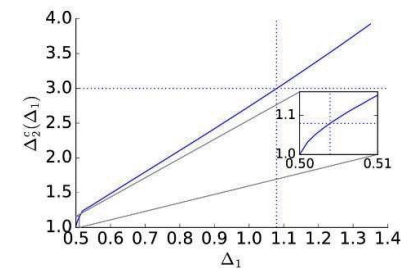
共形ブートストラップによる臨界指数の制限
