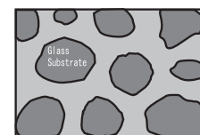
多重連結空間の中では超流動 ^3\text{He} はどうなるのか??
