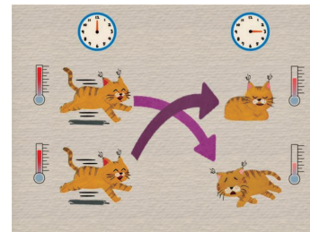
高温状態の量子ドットは低温の系よりも迅速に低温状態へ緩和する。
