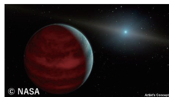
太陽系外の木星型惑星の想像図
