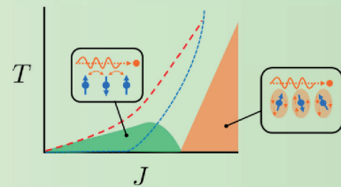
Doniach 相図
