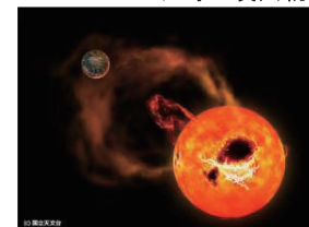
図6 恒星スーパーフレアの噴出物が惑星を襲う概念図
