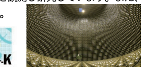
水5万トンを用いた超大型検出器SK SKで観測されたチェレンコフ光
