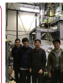
\mu\text{K} の世界のトポロジカル欠陥や量子渦を探索する回転超低温冷凍機
