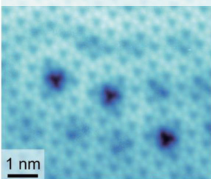
STMによるトポグラフィ像 暗いのは層の欠陥
