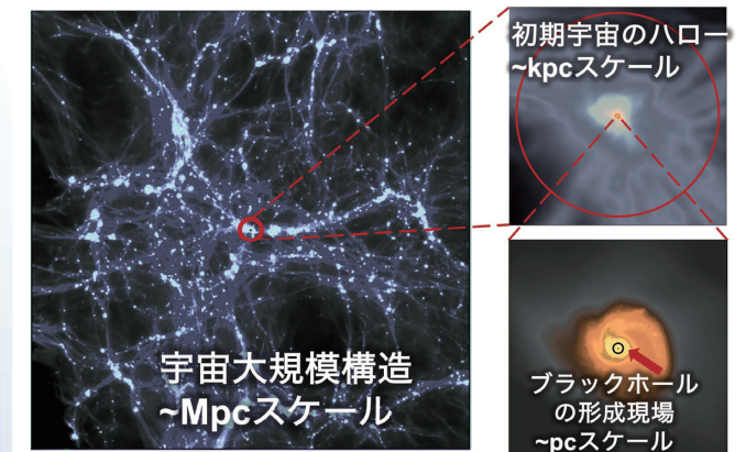
超大質量ブラックホール形成の様子(数値シミュレーション)
