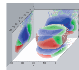
500 \mu\text{K} における核磁気秩序固体 ^4\text{He} の磁区構造 赤青緑に色分けされた独立の磁区が隣り合って存在する様子を MRI 撮影した図と各面への投影図
