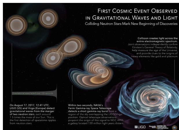
重力波と電磁波の両方が初めて観測された 中性子星連星の合体(GW170817)の模式図
