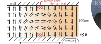
超流動 ^3\text{He} 中でトポロジカルな拘束により安定化されるトポロジカル欠陥が示す新現象
