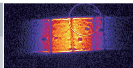
100 \mu\text{m} 厚の平板状の超流動 ^3\text{He} (2mK) の中に発生したトポロジカル欠陥の実空間像を MRI 撮影 (カイラルドメイン実空間観測 Kasai et al. Phys. Rev. Lett. 2018)
