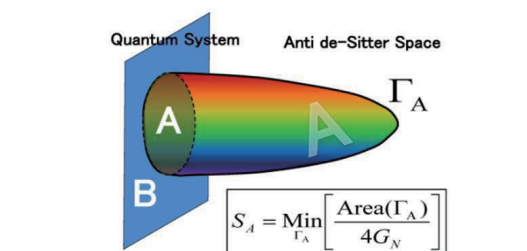
ゲージ重力対応において、量子もつれの量を表すエンタングルメント・エントロピーの幾何学公式と概念図
