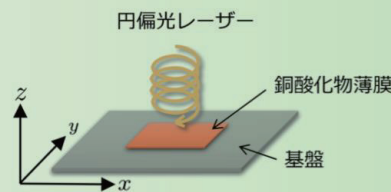
レーザー誘起トポロジカル超伝導の模式図
