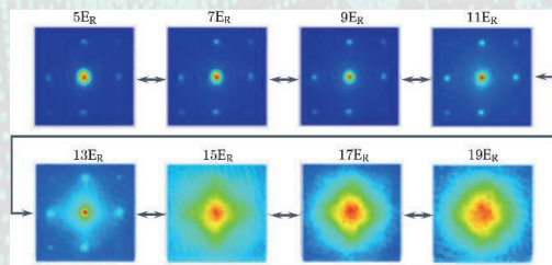
超流動・絶縁体転移の様子。
