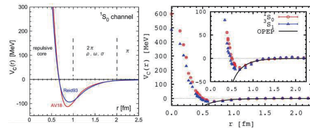
(図1)現象論的核力ポテンシャルの例
