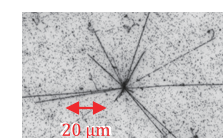
原子核乾板中でのニュートリノ反応
