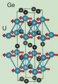
超伝導体UGe 2 の 結晶・磁気構造
