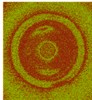
ゲスト分子やイオンの拡散・配位によって、無配向フィルム内部に生じた高分子の(拡散誘起)配向構造のX線回折像
