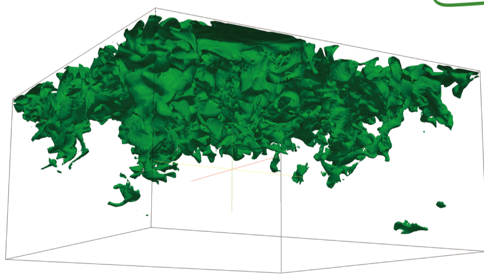
図2: 界面付近での乱流のシミュレーション結果の可視化画像例 吸収された温室効果ガスの濃度場の等値面をひとつ選んで示しています。
