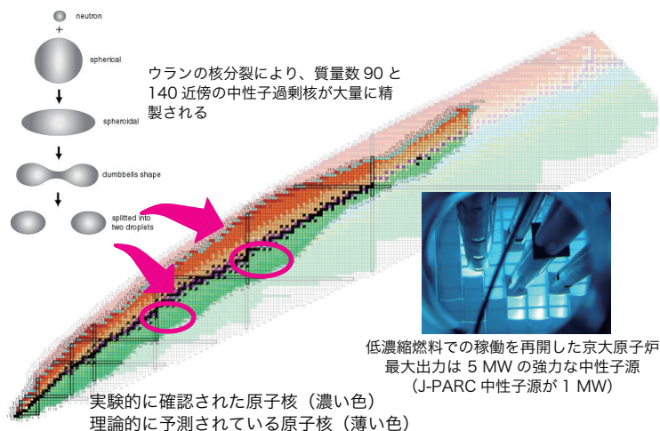
核図表と核分裂による不安定核の生成
