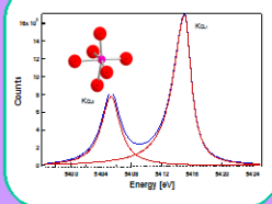
Cr 2 O 3 (八面体至6配位)
