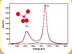
K 2 Cr 2 O 7 (四面体至4配位)
