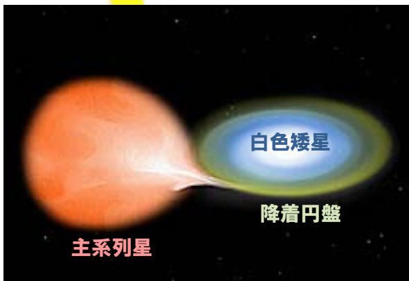
激変星や新星の模式図
