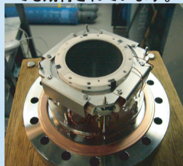
位置敏感型検出器
