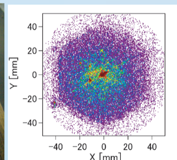
クーロン爆発によるイオンイメージング
