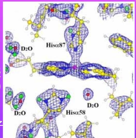
ヒト血液ヘモグロビン分子内で見られた重水素原子(緑で表示)と核密度分布(フーリエ)図
