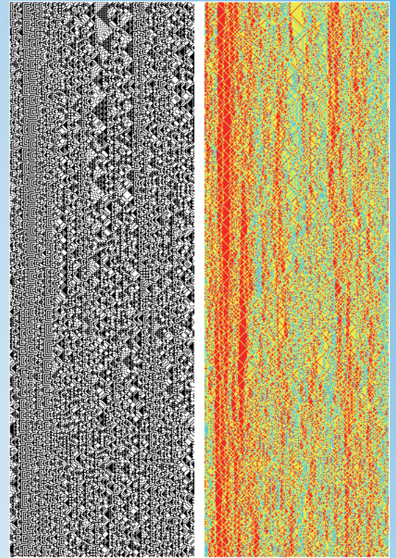
加法的保存量をもつセルオートマトンの時間発展
