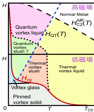
左: Bi (ビスマス) 系 HTSC が示す磁場中相図
