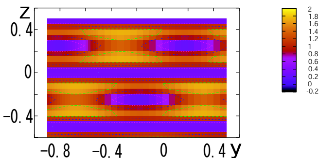
下: 有機超伝導体 \lambda - (\text{BETS})_2\text{FeCl}_4 で実現していると予想される FFLO 相
