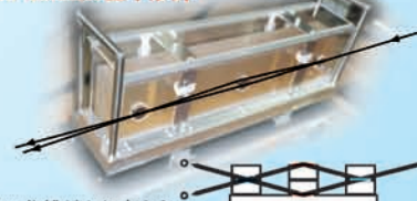
経路の分離がより大きな干渉計で重力が波動関数に与える効果を精密に測定します (COW実験)
